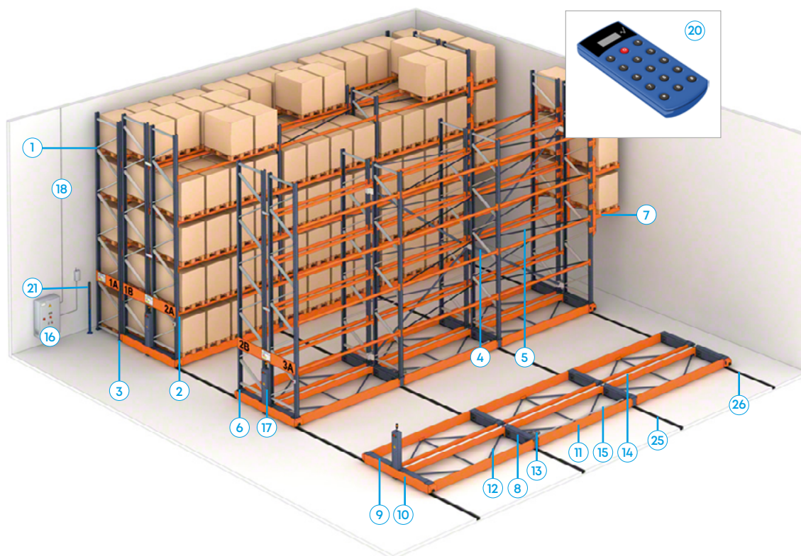
Vodilna tirnica
