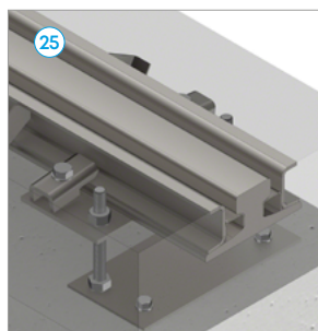
Vodilna tirnica
