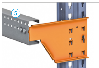
Del C-tirnice
