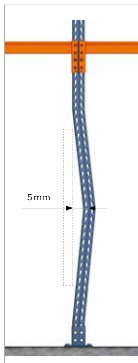
B. Stebri, upognjeni v smeri ravnega dela nosilca, s trajno deformacijo, enako ali večjo od 5 mm, merjeno od središča 1-metrskega intervala.
