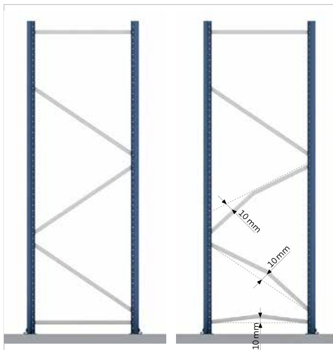
C. Trajne deformacije enake ali večje od 10 mm v vodoravnih in diagonalnih povezavah v kateri koli smeri. Za dolžine, krajše od 1 m, se lahko vrednost 10 mm linearno interpolira.
