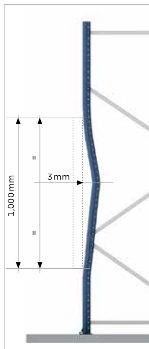
A. Stebri, upognjeni v smeri ravnega dela okvirja, s trajno deformacijo, enako ali večjo od 3 mm, merjeno od središča 1-metrskega intervala.
